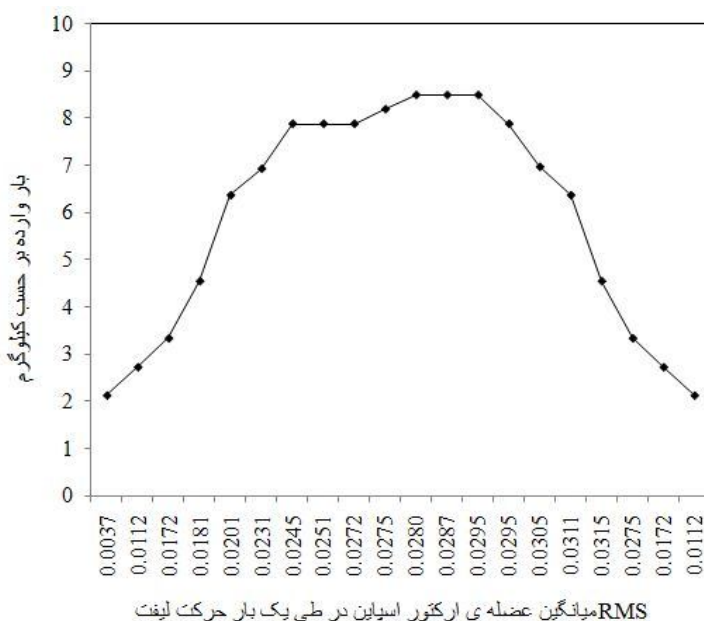
شکل ۳- میزان ریشه‌ی میانگین مجذور گرفته شده از عضله‌ی ارکتور اسپاین نسبت به بار وارده بر فنر تعبیه گشته در پشت لباس کمکی برای برداشتن وزنه
